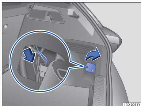
图 121 行李厢内的交流充电插头应急解锁拉索
