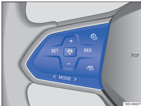
图 93 多功能方向盘左侧：自适应巡航的操作按钮
