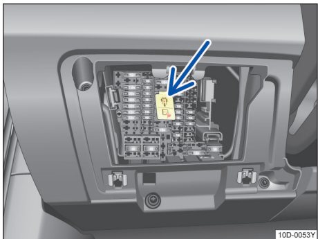
图 128 救援用保险丝
