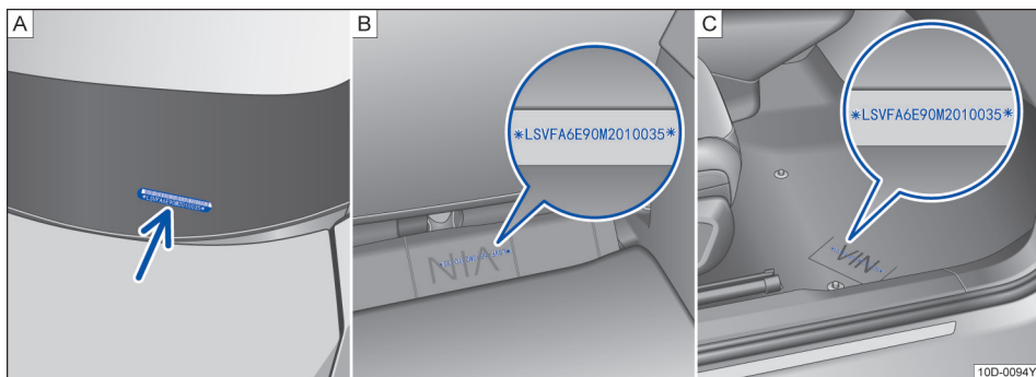
图 146 [A]. 车辆识别代号 [B]. 第二排座椅后侧的车辆识别代号钢印位置 或 [C]. 副驾驶座椅下方的车辆识别代号钢印位置
