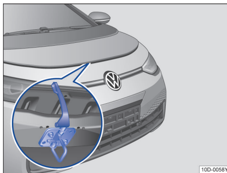
图 135 散热器格栅上方用于打开前舱盖的拉杆
