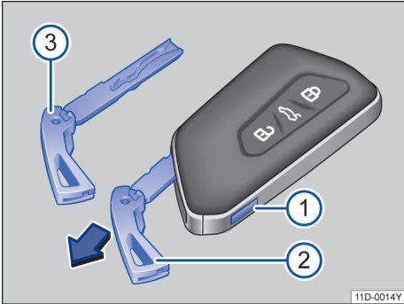
图 39 汽车钥匙：解锁应急钥匙
