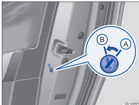
图 49 接通或关闭儿童安全锁
