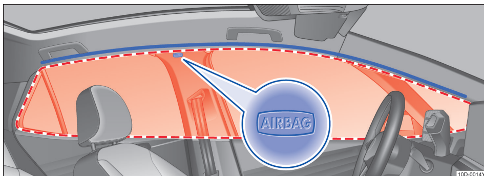
图 31 在汽车左侧：头部安全气囊的安装位置和膨胀范围
