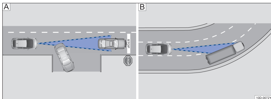
图 91 A. 正在转弯和静止的车辆 B. 弯道行驶
