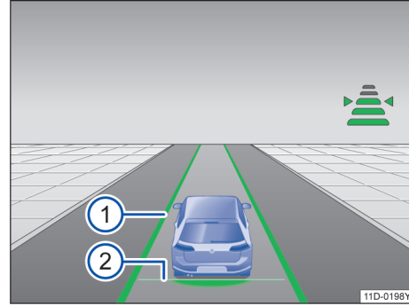
图 97 组合仪表显示屏中：调节激活时显示
