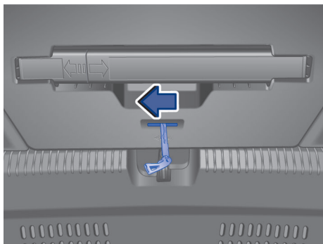
图 52 行李厢盖应急解锁
