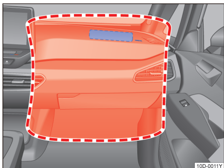
图 28 副驾驶员前部安全气囊的安装位置和膨胀范围
